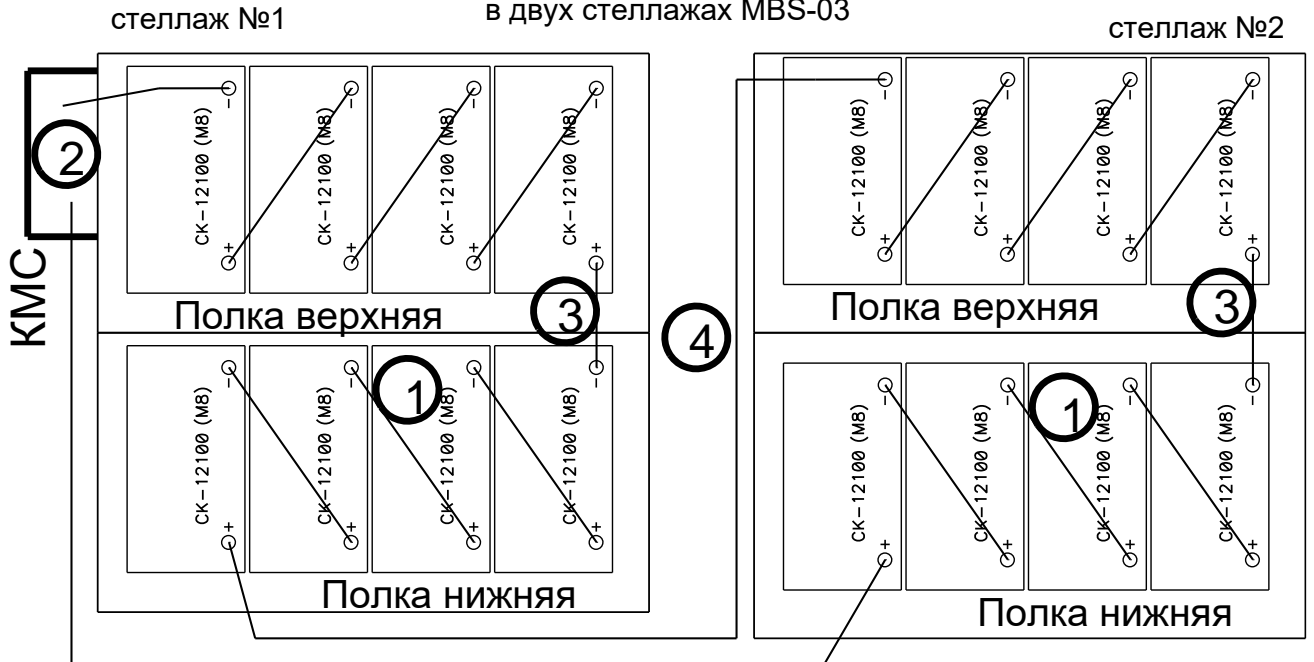
Рисунок 2 – Батарейный комплект S-20-4 для стеллажа МБS-03
